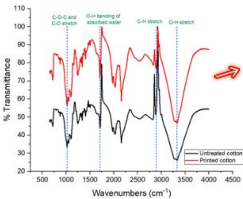
Fig. 1 FTIR Spectra
